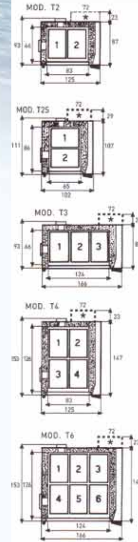
Her İsteğe Cevap Verebilen Soğuk Oda Sistemleri... The Cold Room Systems That Respond Every Demand...
